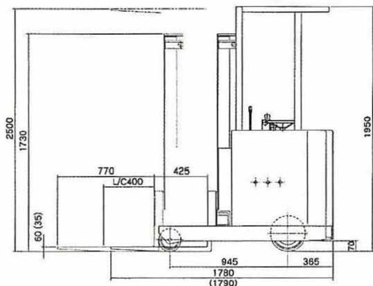
寸法図
